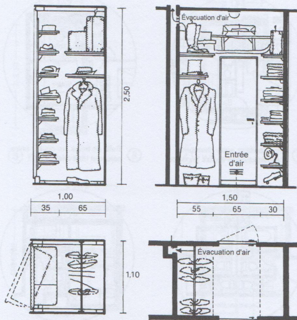
③ Placard double encastré.
