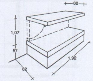
⑫ Lit Pullman pour caravanes et wagons-lits, le dossier relevable constitue un deuxième lit.
