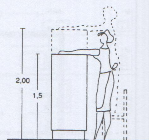
⑧ Hauteurs utiles pour armoire.
