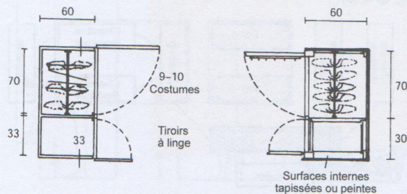
① Placard courant pour vêtements et linge
